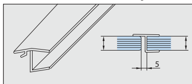
01BTPOLI01 Vinilo perfil h batiente Long: 2.50 m Para cristal: 9.5 y 12.7 mm
