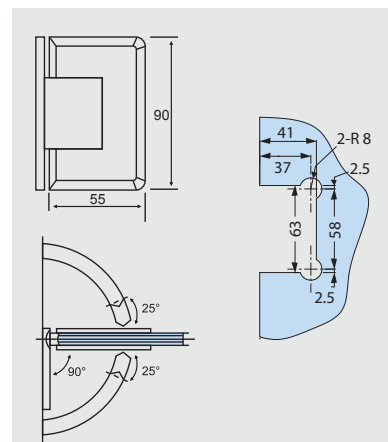
Bisagra muro-cristal montaje simple Zamak Clave: 01BZBISA005
