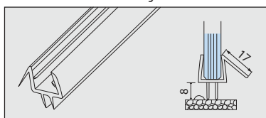
01BTPOLI012 Vinilo botaguas aleta larga con sello al piso Long: 2.50 m Para cristal: 9.5 mm
