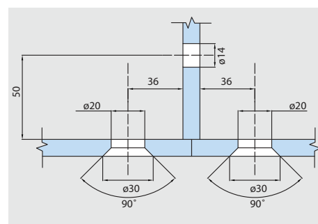
Conector Elite tipo pipa doble para costilla
