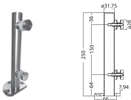
Miniposte Elite de 250 mm con brida Clave: 01ETCONE031
