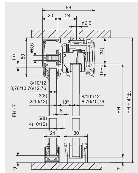
MONTAJE CON PANEL FUO
