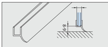
01BTPOLI00 Vinilo aleta suave Long: 2.50 m Para cristal: 6 mm, 9.5 mm y 12.7 mm
