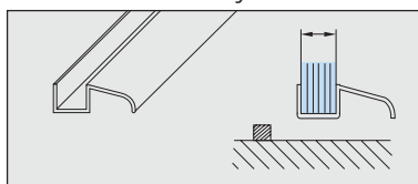
01BTPOLI011 Vinilo botaguas Long: 2.50 m Para cristal: 9.5 mm
