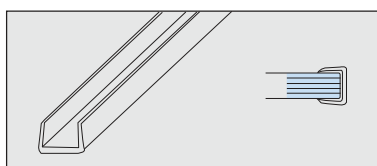
01BTPOLI0 Vinilo convertidor Long: 2.50 m De 6 mm a 9 mm De 9 mm a 12 mm
