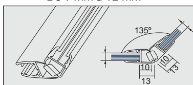
01BTPOLI023 Vinilo magnético 135° (juego de 2 tramos) Long: 2.50 m Para cristal: 9.5 mm
