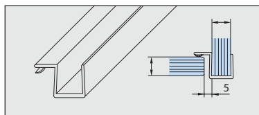
01BTPOLI01 Vinilo perfil k batiente Long: 2.50 m Para cristal: 9.5 y 12.7 mm
