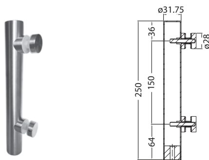
Miniposte Elite de 250 mm sin brida Clave: 01ETCONE032
