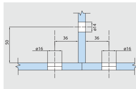
Conector Elite tipo pipa doble para costilla con tapas
